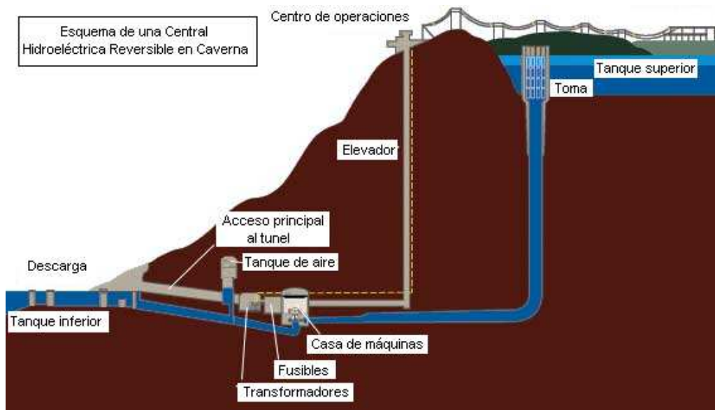
Central hidroeléctrica de bombeo. Imagen de Alfredobi en Wikipedia bajo Dominio Público.
